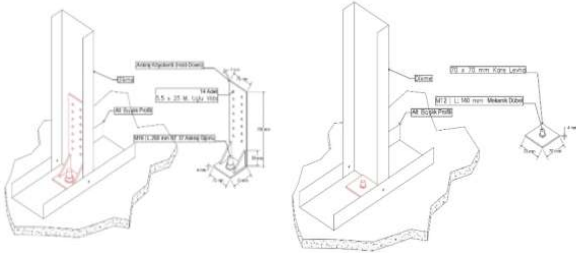
Şekil 3. Kimyasal ankraj detayı (Bekçi,2025) Şekil 4. Mekanik ankraj detayı (Bekçi,2025)
