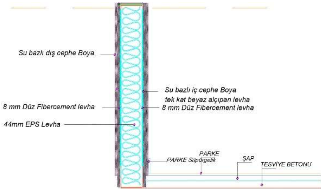
Şekil 1. Pres Panel duvar detayı (Bekçi,2025)
