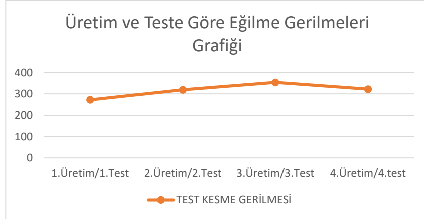
Grafik 4.Üretim ve Teste Göre Eğilme Gerilmeleri Grafığı
