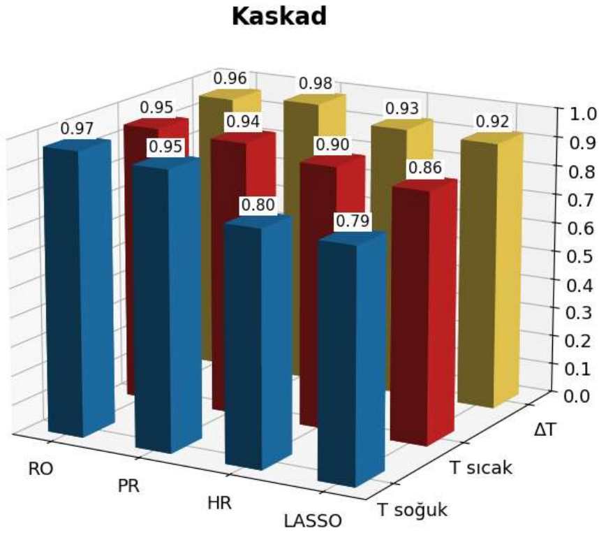
Şekil 10. KRHVT deney seti T_{\text{sıcak}} , T_{\text{soğuk}} ve \Delta T ML yöntemlerine ait testlerin R^2 grafiği
