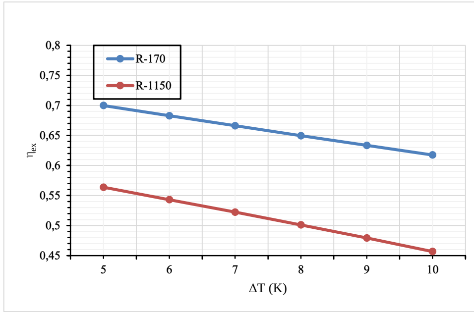
Şekil 5. Ekserji veriminin KID sıcaklık farkıyla değişimi
