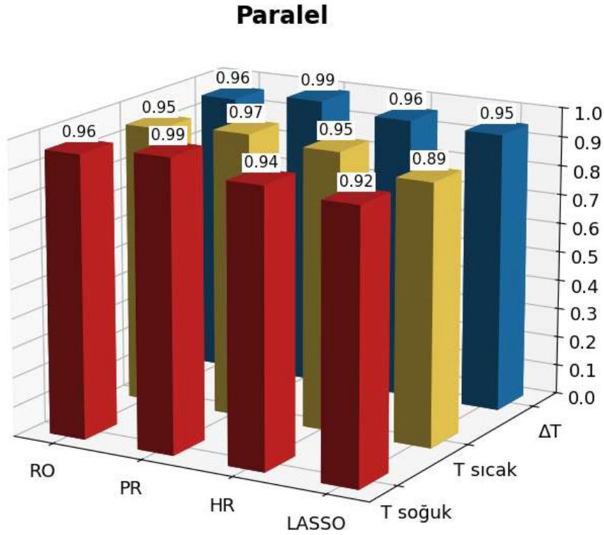
Şekil 9. PRHVT deney seti T_{\text{sıcak}} , T_{\text{soğuk}} ve \Delta T ML yöntemlerine ait testlerin R^2 grafiği
