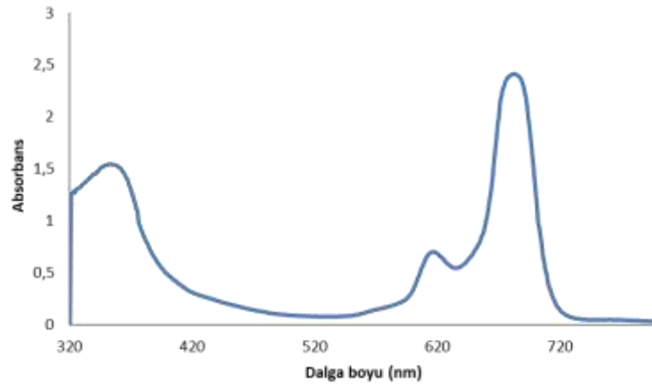
Şekil 4. Ftalosiyenin bileşiğinin UV-Vis ( 10^{-5} M, DMSO) spektrumu
