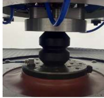
Şekil 3. (a) M+P International Yüksek Frekans Dinamik Test Cihazı (b) Kauçuk Takoz Test Numunesi
