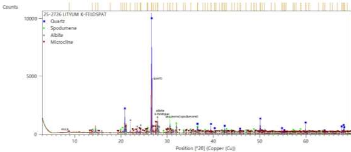
Görsel 2. Lityum Feldspat Numunesinin Mineralojik Analizi.
