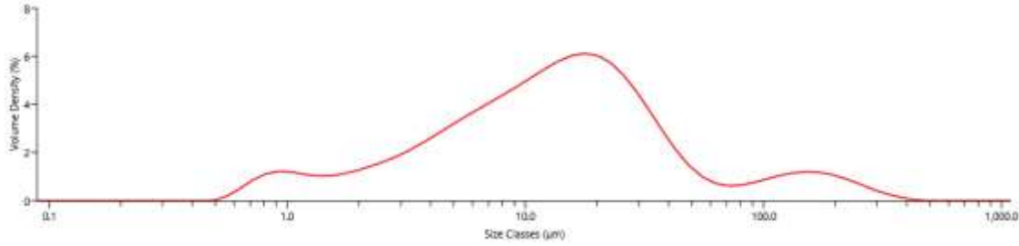
Görsel 1. Tedarik Edilen Lityum Feldspat Numunesinin Tane Boyut Dağılım Grafiği.
