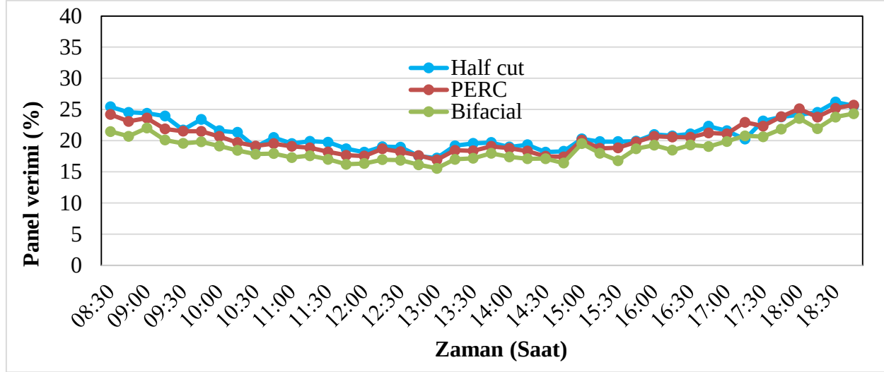
Şekil 3. Zamana bağlı panel verimlerinin değişimi (0° eğim- yön 180°)
