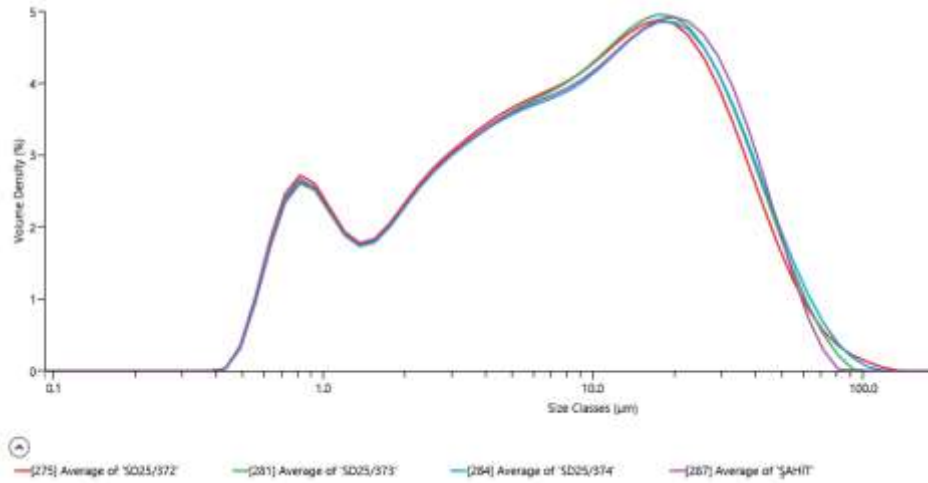
Görsel 3. Hazırlanan Sırların Tane Boyut Dağılım Grafiği.
