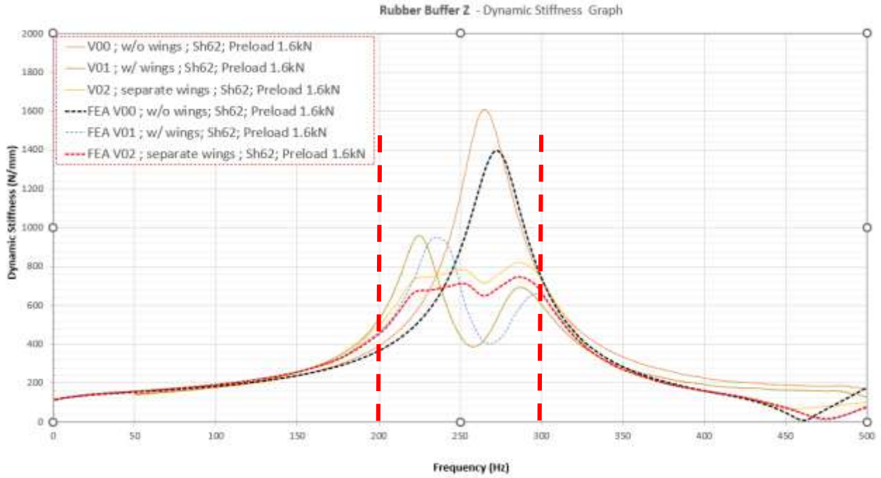
Şekil 9. V00, V01 ve V02 geometrilerine ait sanal prototip (FEA) ve fiziki parçaların karşılaştırmalarında, 500 Hz'e kadar dinamik rijitlik değişimleri
