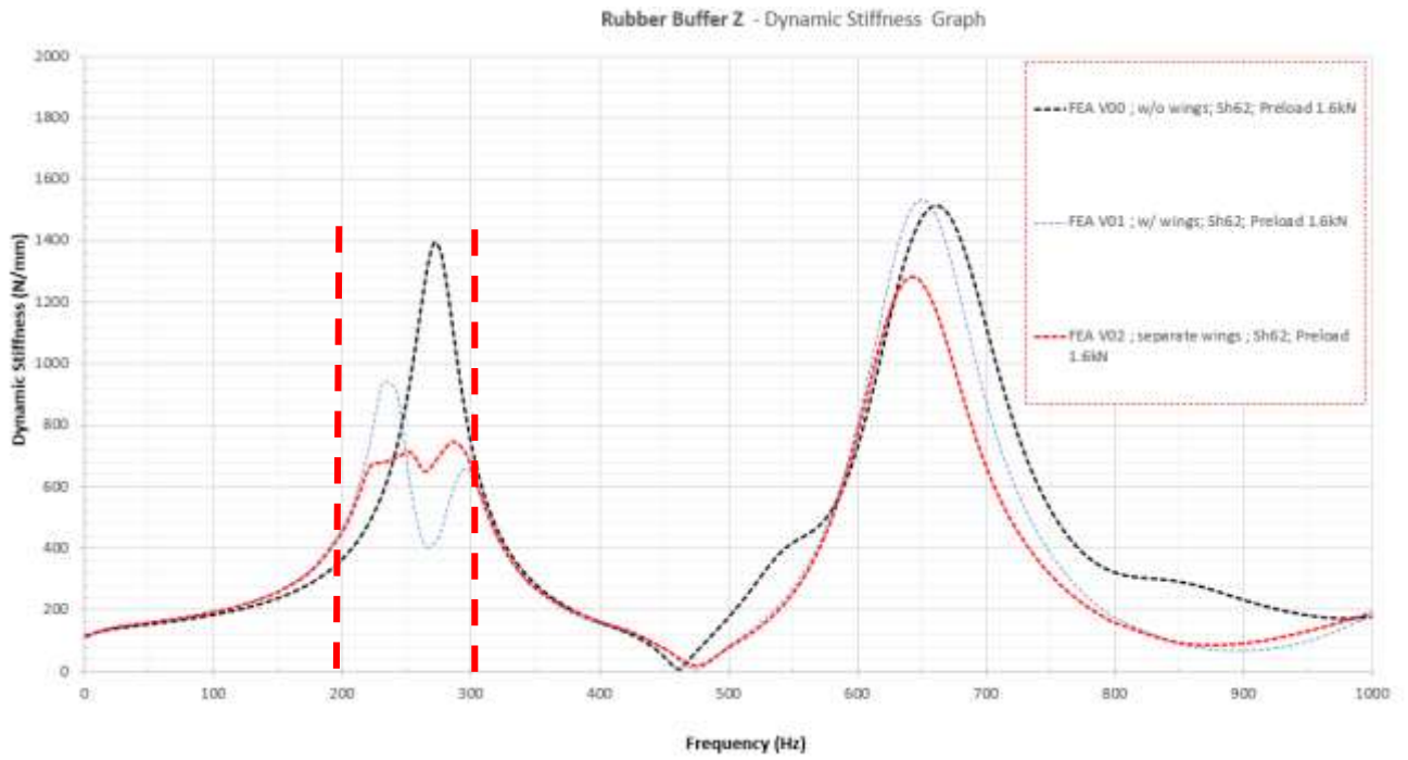
Şekil 5. V00, V01 ve V02 geometri tasarımlarına ait sanal prototiplerin FEA ile elde edilen dinamik rijitlik (stiffness) değerlerinin, 0–1000 Hz frekans aralığında karşılaştırılması
