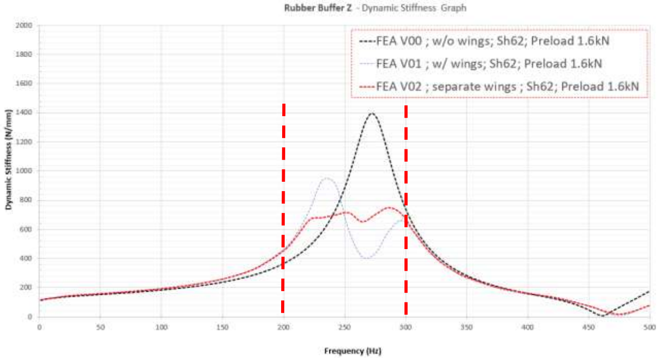
Şekil 6. V00, V01 ve V02 geometrilerine ait parçaların FEA dayalı karşılaştırmalarında, 500 Hz'e kadar dinamik rijitlik değişimleri
