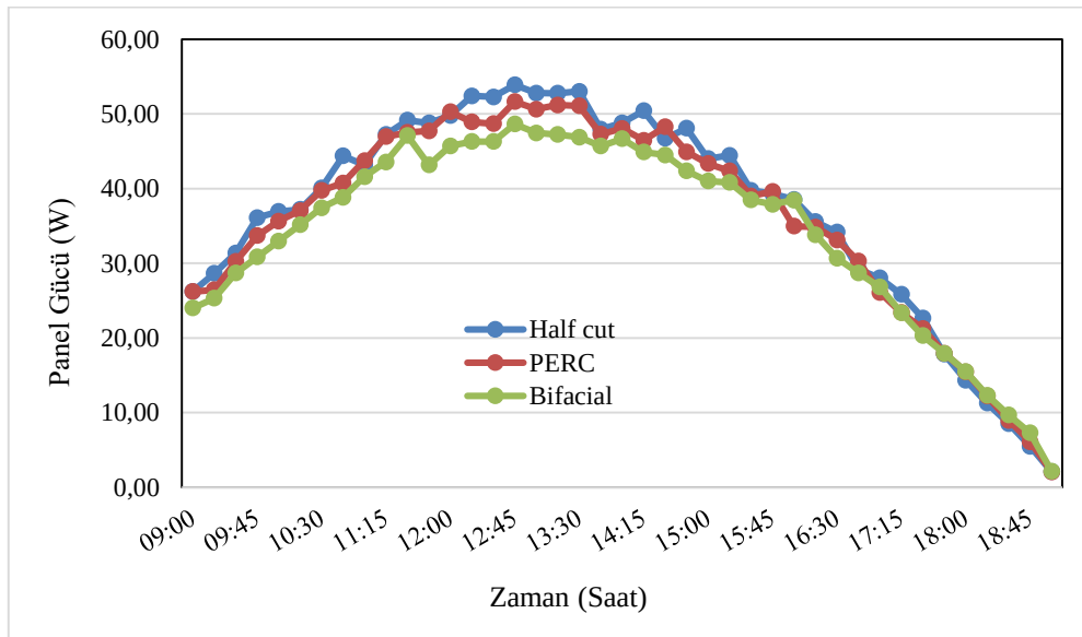
Şekil 4. Zamana bağlı panel güçlerinin değişimi (25° eğim- yön 180°)
