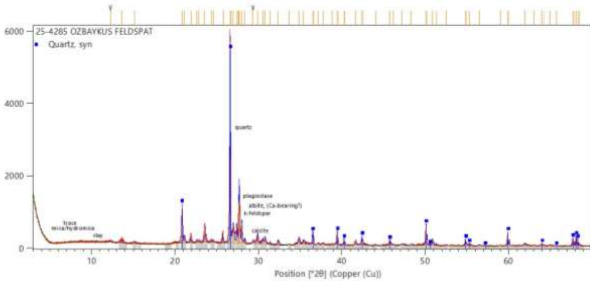
Görsel 2. Adıyaman Felspat Numunesine Ait Mineralojik Analizi.
