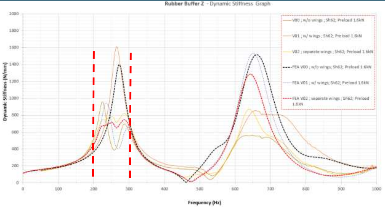
Şekil 8. V00, V01 ve V02 geometri tasarımlarına ait sanal prototip ve fiziki parçalardan elde edilen dinamik rijitlik (stiffness) değerlerinin, 0–1000 Hz frekans aralığında karşılaştırılması
