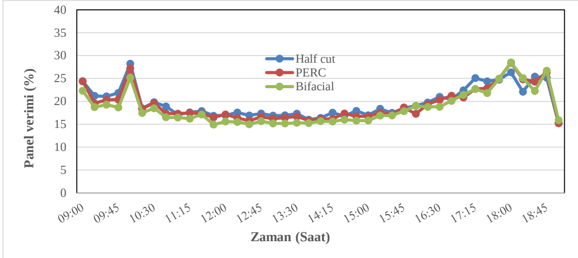
Şekil 5. Zamana bağlı panel verimlerinin değişimi (25 eğim- yön 180°)
