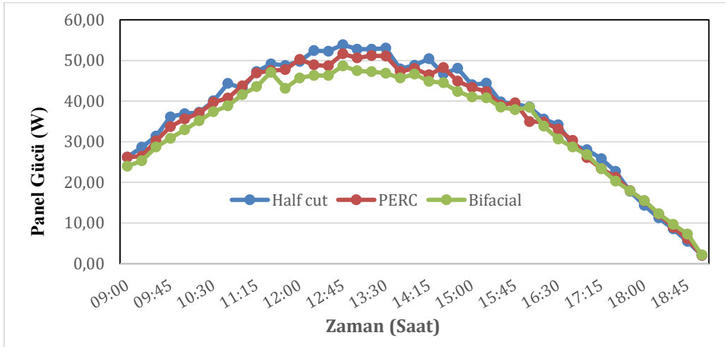
Şekil 2. Zamana bağlı panel güçlerinin değişimi (0° eğim- yön 180°)
