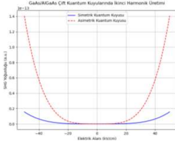
Şekil 1: Simetrik (düz çizgi) ve asimetrik (kesikli çizgi) GaAs/AlGaAs çift kuantum kuyularında elektrik alanına bağlı SHG yoğunluğu.
